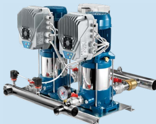
2P + VSD
